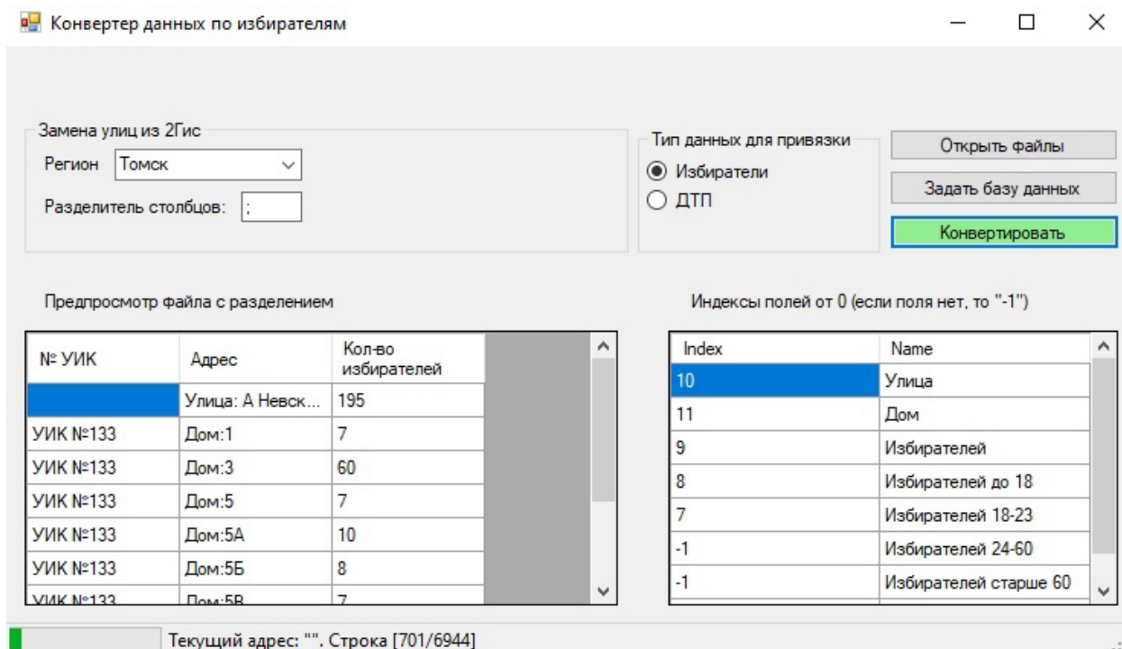
Рисунок 3 – Конвертация исходных данных в базу данных в программном продукте VoterDataConverterR
